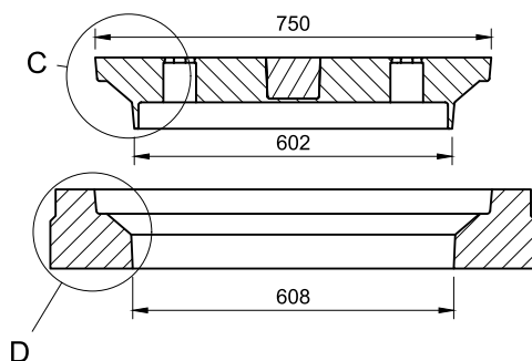
A-A (1:8)
